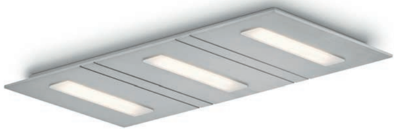
SINA-3 91.354.05 mattnickel 3 x 13,6 W LED, 5.250 lm, 2.200 - 2.900 K, Ra > 90 Energieeffizienzklasse A+ flacher Aufbau durch Magnethalterung zentral dimmbar über Universal Triac LED Dimmer 2-100 W mit dim to warm Technologie
